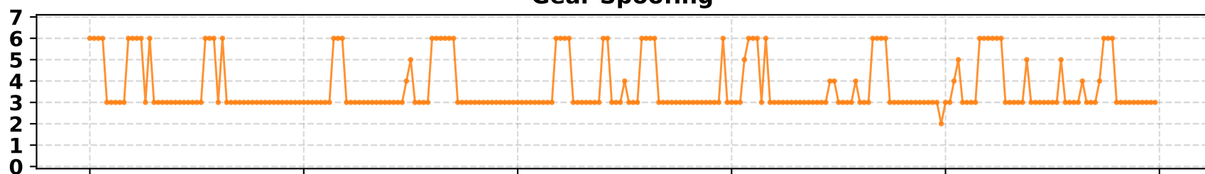
Malfunction
